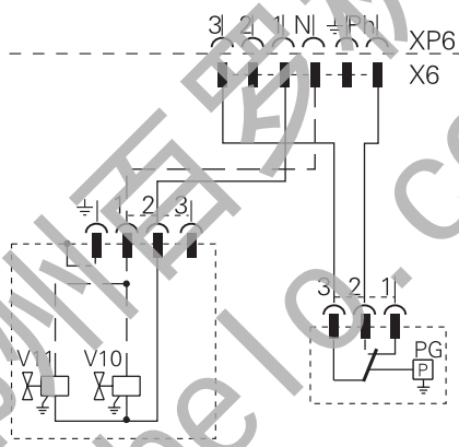
燃气阀组接线
